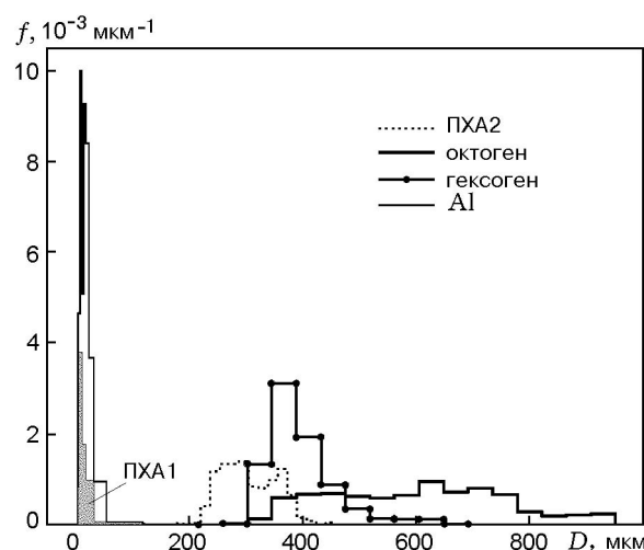
Рис. 1. Гранулометрический состав порошкообразных компонентов топлив:
