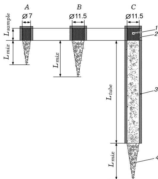
Рис. 3. Варианты геометрии опытов для изменения времени пребывания агломератов в пламени:
