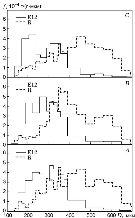
Рис. 7. Массовые распределения агломератов топлив E12 и R в диапазоне размеров 100 ÷ 700 мкм при вариации геометрии опытов:
