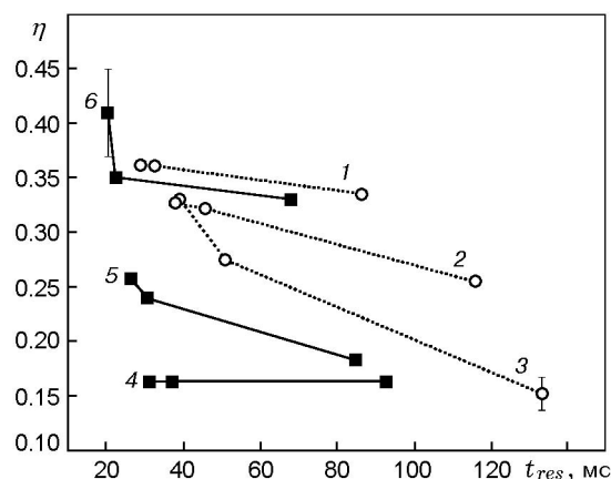
Рис. 6. Динамика выгорания алюминия из совокупности агломератов топлив E12 и R: зависимости неполноты сгорания алюминия \eta от времени пребывания t_{res} :
