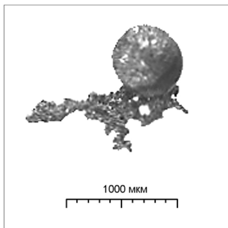
Рис. 8. Агломерат с примыкающими образованиями из полуспеченных частиц металла, обеспечивающими его удержание на поверхности горения:
