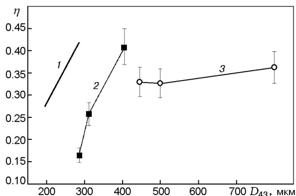
Рис. 9. Зависимость неполноты сгорания алюминия от размера агломератов:
