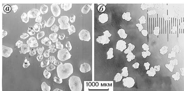
Рис. 2. Вид частиц октогена (а) и гексогена (б) фракции 250 ÷ 700 мкм
