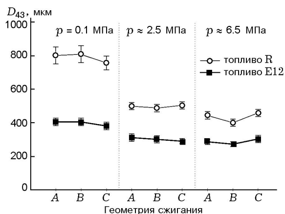
Рис. 5. Сравнение средних размеров D_{43} агломератов топлив E12 и R, отобранных при вариации давления и геометрии сжигания
