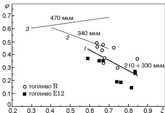
Рис. 10. Влияние размера агломератов на зависимость \varphi(\xi) :
