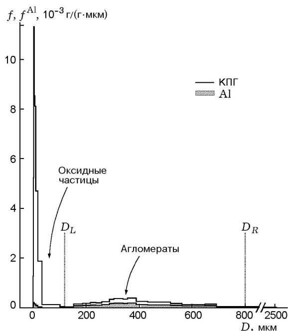
Рис. 4. Массовые распределения КПГ и несгоревшего алюминия в КПГ (затемненная область) по размерам в диапазоне от 0.5 мкм до максимального:
