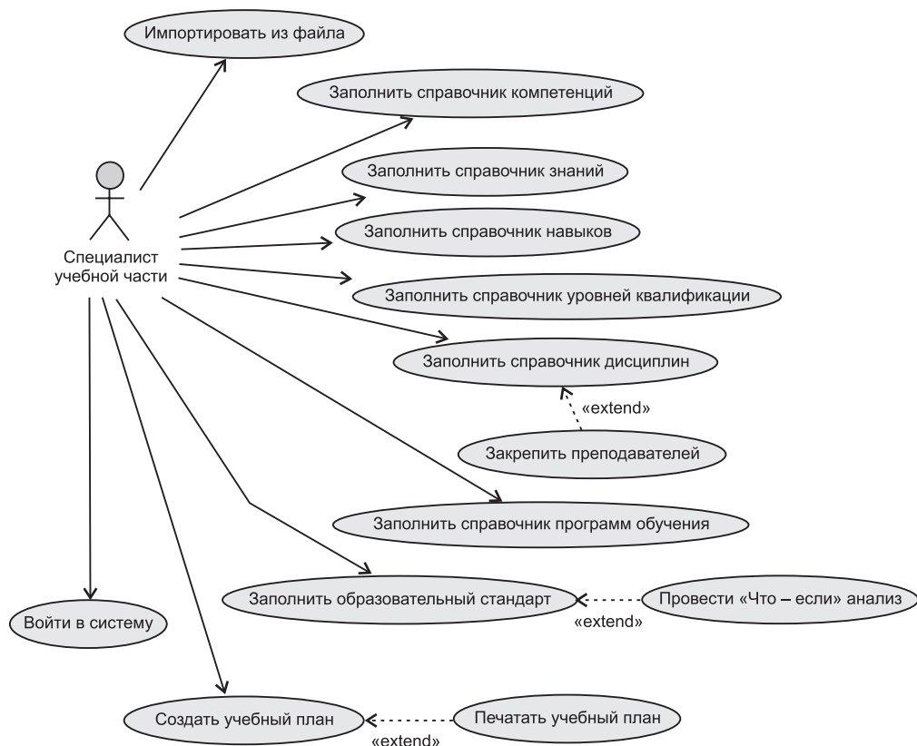
Рис. 7. Прецеденты системы для специалиста учебной части
