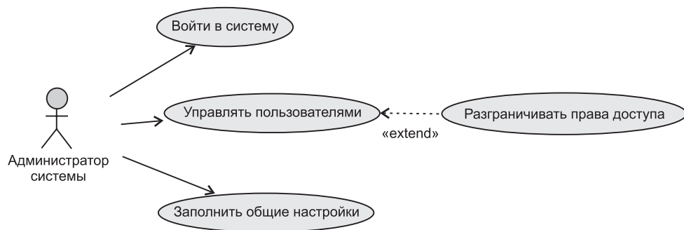
Рис. 11. Прецеденты системы для администратора
