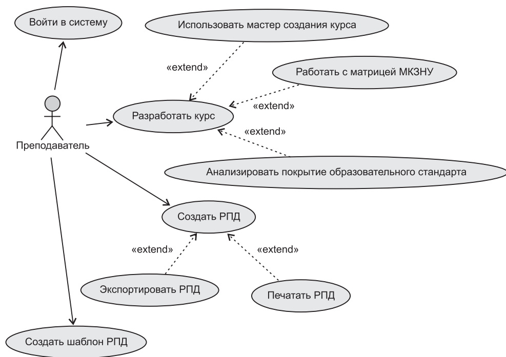
Рис. 8. Прецеденты системы для преподавателя
