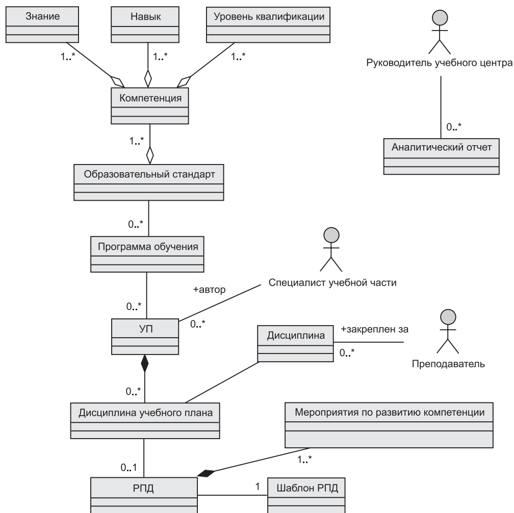
Рис. 6. Модель предметной области системы
