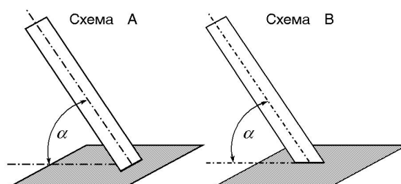
Рис. 1. Схемы ориентации подложек в пространстве
