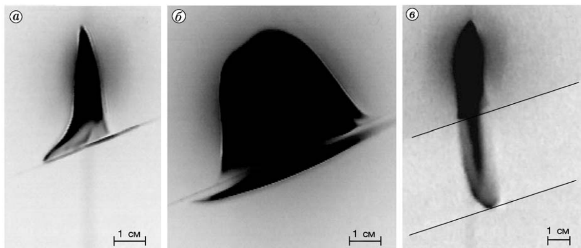
Рис. 2. Видеокadres распространения пламени додекана снизу вверх по верхней (а) и нижней (б) поверхностям подложки при \alpha = 22.6^\circ и по боковой поверхности (в) при \alpha = 20^\circ :
