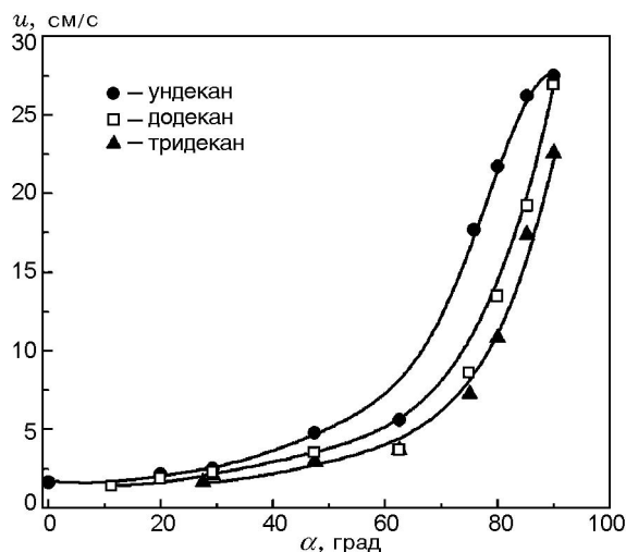
Рис. 8. Зависимости скорости распространения пламени по одной стороне подложки от угла \alpha для различных топлив:
