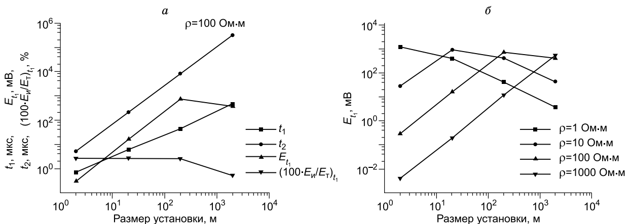
Рис. 7. Параметры, зависящие от размера установки ( a ), и графики зависимости уровня сигнала в точке t_1 от размера установки на разных разрезах ( b ).
