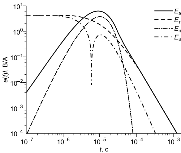
Рис. 4. Составляющие измеряемого сигнала.
