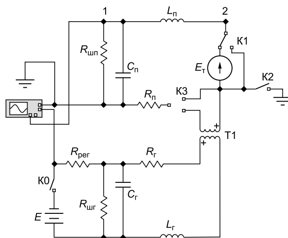
Рис. 1. Эквивалентная электрическая схема генераторно-приемной установки для нестационарного электромагнитного зондирования.
