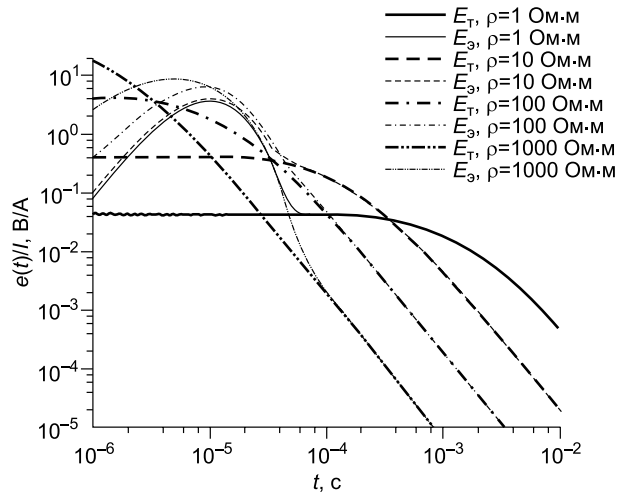
Рис. 2. Теоретические ( E_T ) и псевдоэкспериментальные сигналы ЭДС ( E_3 ) разных разрезов, рассчитанные для установки 200 м.
