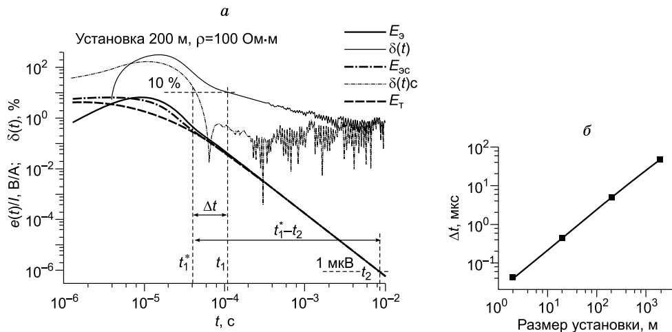
Рис. 3. Пример определения сдвига сигнала по времени \Delta t и границ доверия t_1 и t_2 (а) и кривая зависимости величины сдвига от размера установки (б).
