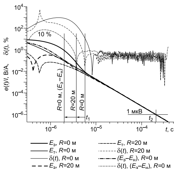
Рис. 10. Уменьшение прямой наводки выносом приемника за пределы излучателя.
