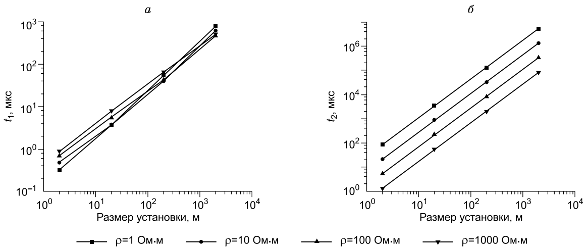
Рис. 6. Зависимость параметров t_1 ( a ) и t_2 ( b ) от размера установки и удельного сопротивления среды.
