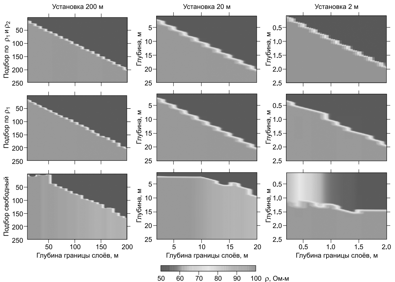
Рис. 9. Геоэлектрические двухслойные разрезы с равномерным погружением основания.
