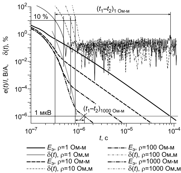
Рис. 8. Границы доверия для псевдоэкспериментальных сигналов от разных разрезов на примере установки 2 м.
