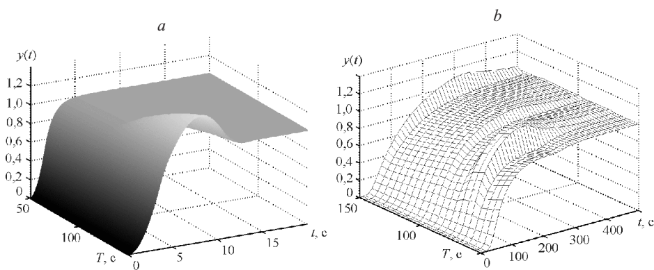
Рис. 4. Динамика изменения переходного процесса в системе при действии параметрического возмущения: для объекта без запаздывания (а); для объекта, обладающего транспортным запаздыванием (б)
