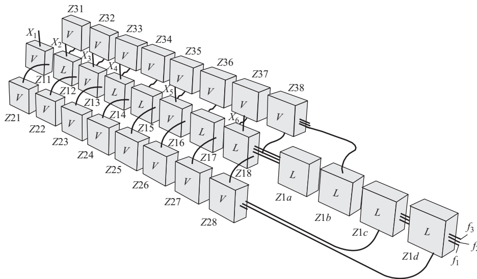
Рис. 2. Квазиизотропная среда
