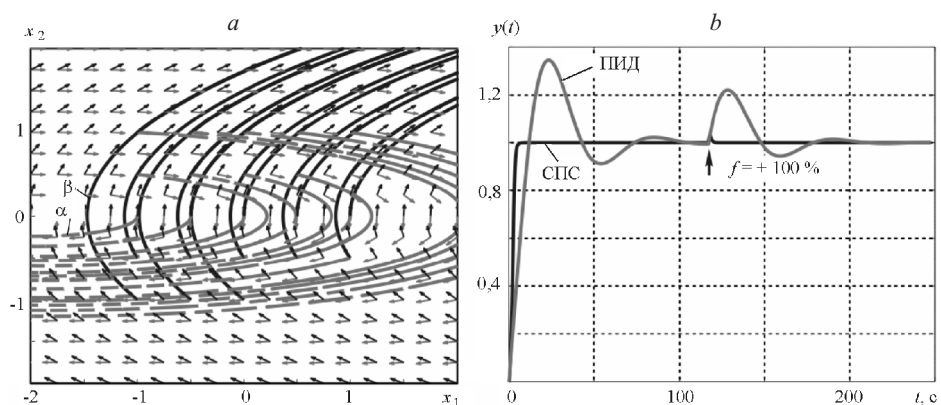
Рис. 3. Результаты моделирования: фазовые портреты и поля направлений для линейных структур (а); динамические характеристики рассматриваемой автоматической системы регу-
