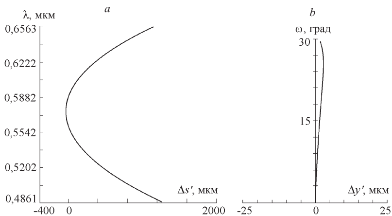
Рис. 3. Кривые остаточных хроматических aberrаций: хроматизм положения (а), хроматизм увеличения (б)
