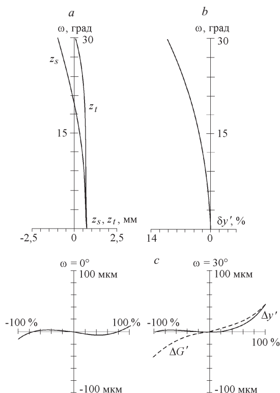
Рис. 2. Кривые остаточных монохроматических aberrаций: астигматизм и кривизна поля (а); дисторсия (b); aberrации широких наклонных пучков ( y для меридиональной плоскости, G для сагиттальной плоскости) (с)
