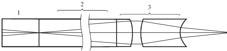
Рис. 1. Оптическая схема иглообразной части жесткого эндоскопа, включающей градан-объектив (1), градан-транслятор (2) и двухлинзовый корректор аберраций (3)
