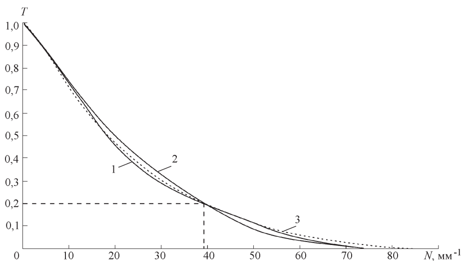
Рис. 4. Дифракционная полихроматическая частотно-контрастная характеристика: при N = 0 (кривая 1); при N = 30 для меридиональной (2) и сагиттальной (3) плоскостей
