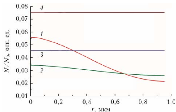
Рис. 7. Распределения концентрации электронов в частице порошка в различные моменты времени: 1 — 0,1 \text{ нс} ; 2 — 0,15 \text{ нс} ; 3 — 0,5 \text{ мкс} ; 4 — 1 \text{ мкс} (см. цветной рисунок на сайте http://iao.ru/ru/content/vol.37-2024/iss.04 )
