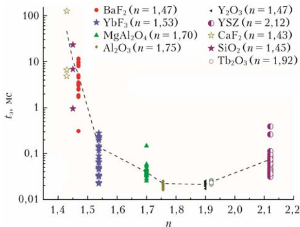
Рис. 1. Зависимость времени задержки t_3 появления лазерного факела от показателя преломления n для различных пористых материалов (из прессованного порошка) при интенсивности излучения волоконного лазера I = 0,46 \text{ МВт/см}^2 [9] (см. цветной рисунок на сайте http://iao.ru/ru/content/vol.37-2024/iss.04 )
