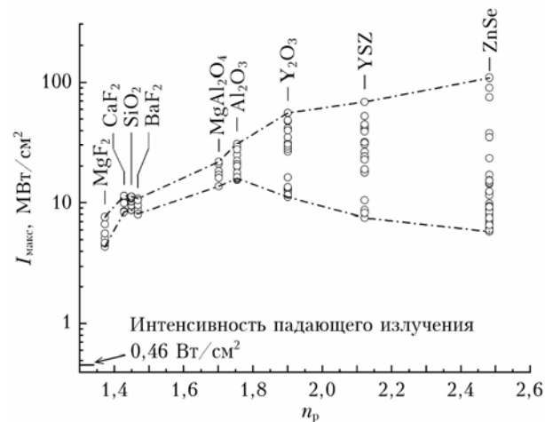
Рис. 3. Зависимость максимальной интенсивности излучения от показателя преломления материала с учетом ширины спектральной линии для волоконного иттербиевого лазера ( \lambda = 1070 \pm 3,2 \text{ нм} )
