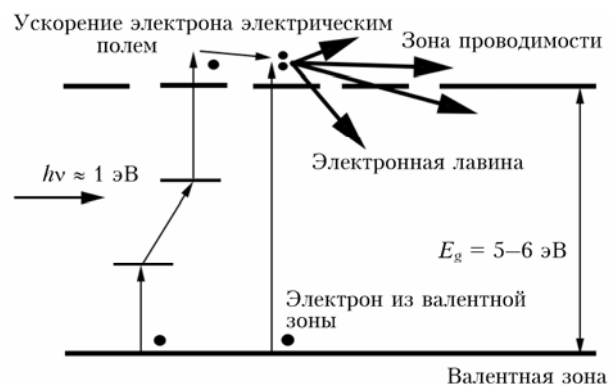
Рис. 4. Механизм инициирования нагрева прессованной мишени в области локального максимума интенсивности излучения
