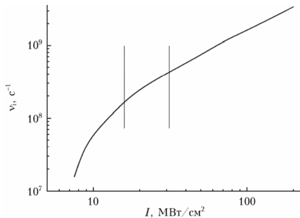
Рис. 6. Зависимость частоты ионизации от интенсивности лазерного излучения для \text{Al}_2\text{O}_3
