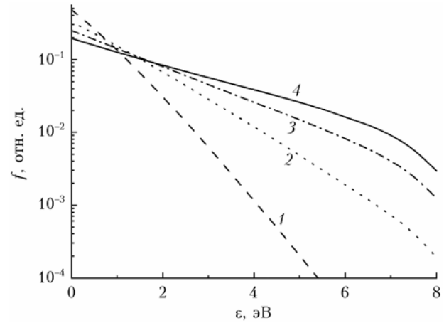
Рис. 5. Нормированная функция распределения электронов по энергии для Al_2O_3 в различные моменты времени: 1 — 0,4 нс; 2 — 1 нс; 3 — 2 нс; 4 — 10 нс. На оси энергии 0 соответствует дну зоны проводимости
