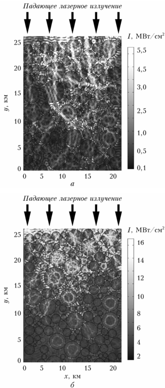
Рис. 2. Распределение интенсивности излучения волоконного лазера в прессованном порошке из \text{Y}_2\text{O}_3 ( n_p = 1,90 ) (а) и \text{ZnSe} ( n_p = 2,48 ) (б) при интенсивности падающего излучения 0,46 \text{ MBt/cm}^2
