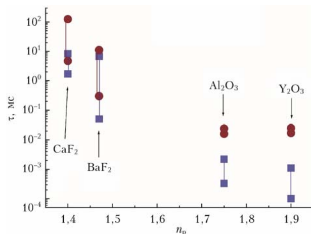
Рис. 8. Зависимости расчетного характерного времени ионизации в частице порошка диэлектрика (квадраты) и времени формирования лазерного факела, измеренного экспериментально (круги), от показателя преломления диэлектрика (см. цветной рисунок на сайте http://iao.ru/ru/content/vol.37-2024/iss.04 )
