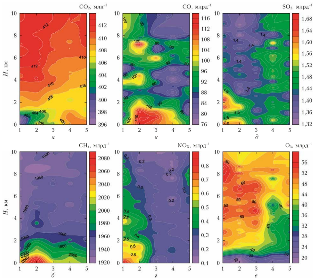
Рис. 2. Вертикальное распределение концентрации малых газовых составляющих над морями Российского сектора Арктики: а – \text{CO}_2 ; б – \text{CH}_4 ; в – \text{CO} ; г – \text{NO}_x ; д – \text{SO}_2 ; е – \text{O}_3 . Здесь и на рис. 4 цифры на оси x: 1 – Баренцево море, 2 – Карское море, 3 – море Лаптевых, 4 – Восточно-Сибирское море, 5 – Чукотское море
