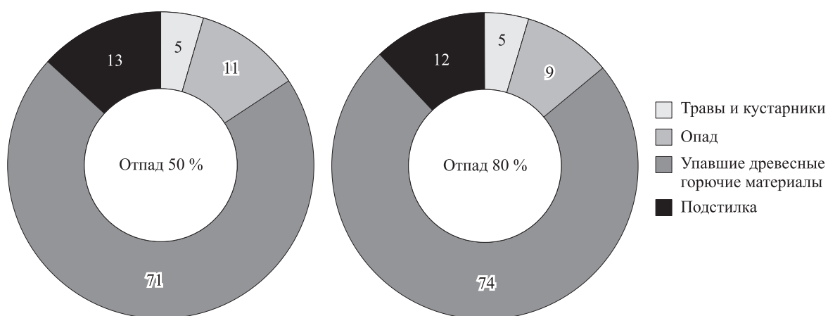
Рис. 4. Структура запасов лесных горючих материалов в темных хвойных насаждениях с разной степенью нарушения, %.
