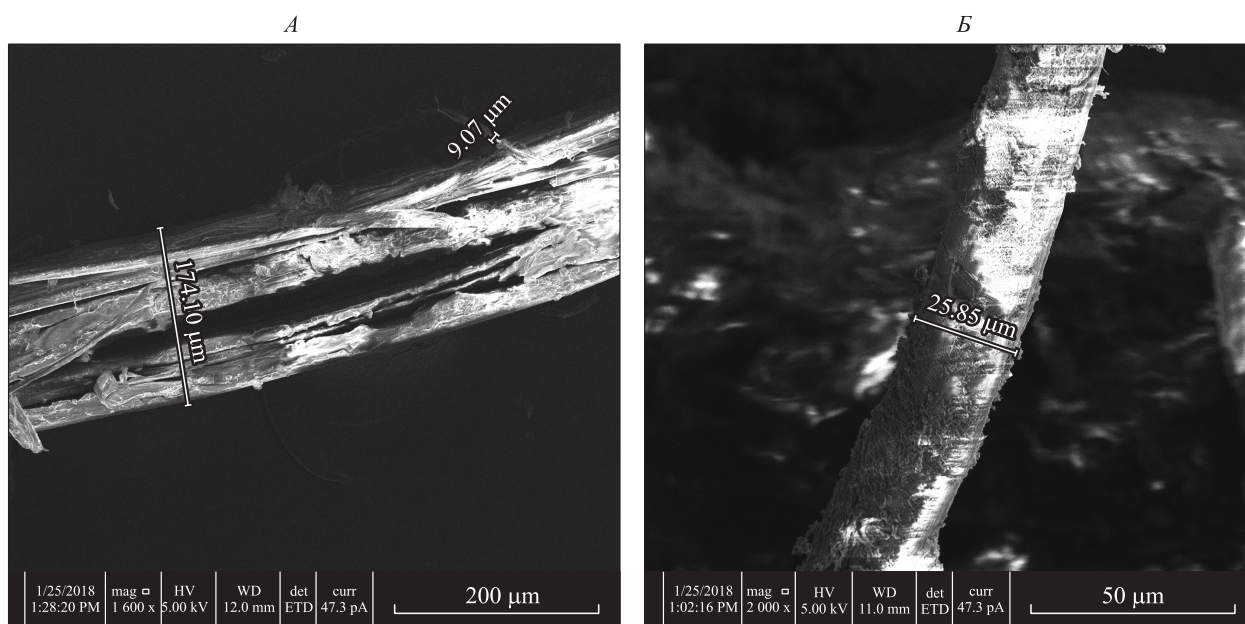
Рис. 3. Микроструктура льняных отходов: А – поврежденное волокно, Б – волокно с осажженным наполнителем.
