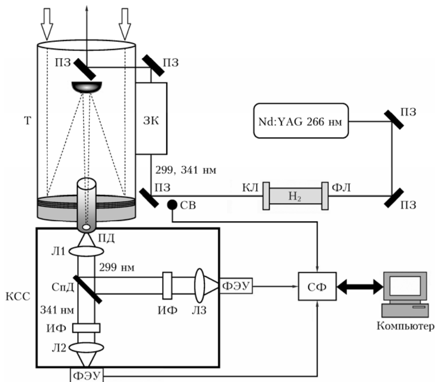
Рис. 1. Блок-схема мобильного озонного лидара: Nd:YAG — твердотельный лазер; ФЛ — фокусирующая линза; КЛ — коллимирующая линза; Н 2 — ячейка вынужденного комбинационного рассеяния с водородом, оборудованная линзами; ПЗ — поворотное зеркало; ЗК — зеркальный коллиматор; Т — приемный телескоп, собранный по схеме Кассегрена с главным зеркалом диаметром 0,35 м; КСС — кювета спектральной селекции, оборудованная линзами; ПД — поляризатор; Л — линза; СпД — спектроделительное зеркало; ИФ — интерференционные фильтры; ФЭУ — модуль фотоэлектронного умножителя H12386-210 HAMAMATSU; СФ — счетчик фотонов PHCOUNT_4E; СВ — световод для запуска счетчика фотонов; Компьютер — персональный компьютер для сбора и хранения получаемой информации
