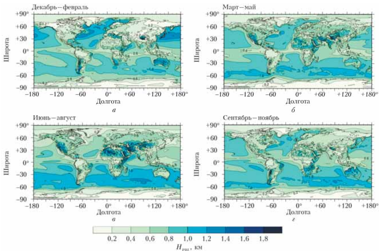
Рис. 1. Осредненная за 2003–2020 гг. среднесезонная высота верхней границы ППС относительно поверхности Земли зимой (а), весной (б), летом (в) и осенью (г) (цв. рисунок см. http://iao.ru/ru/content/vol.35-2022/iss.07 )
