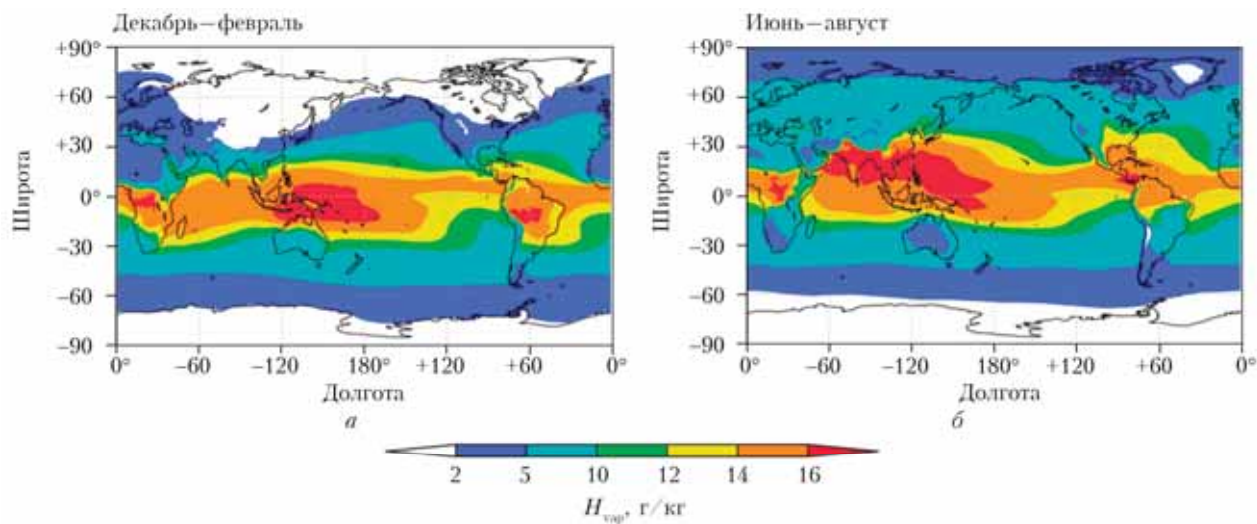
Рис. 7. Среднесезонные значения удельной влажности зимой (а) и летом (б) на изобарическом уровне 950 гПа по данным реанализа ERA5
