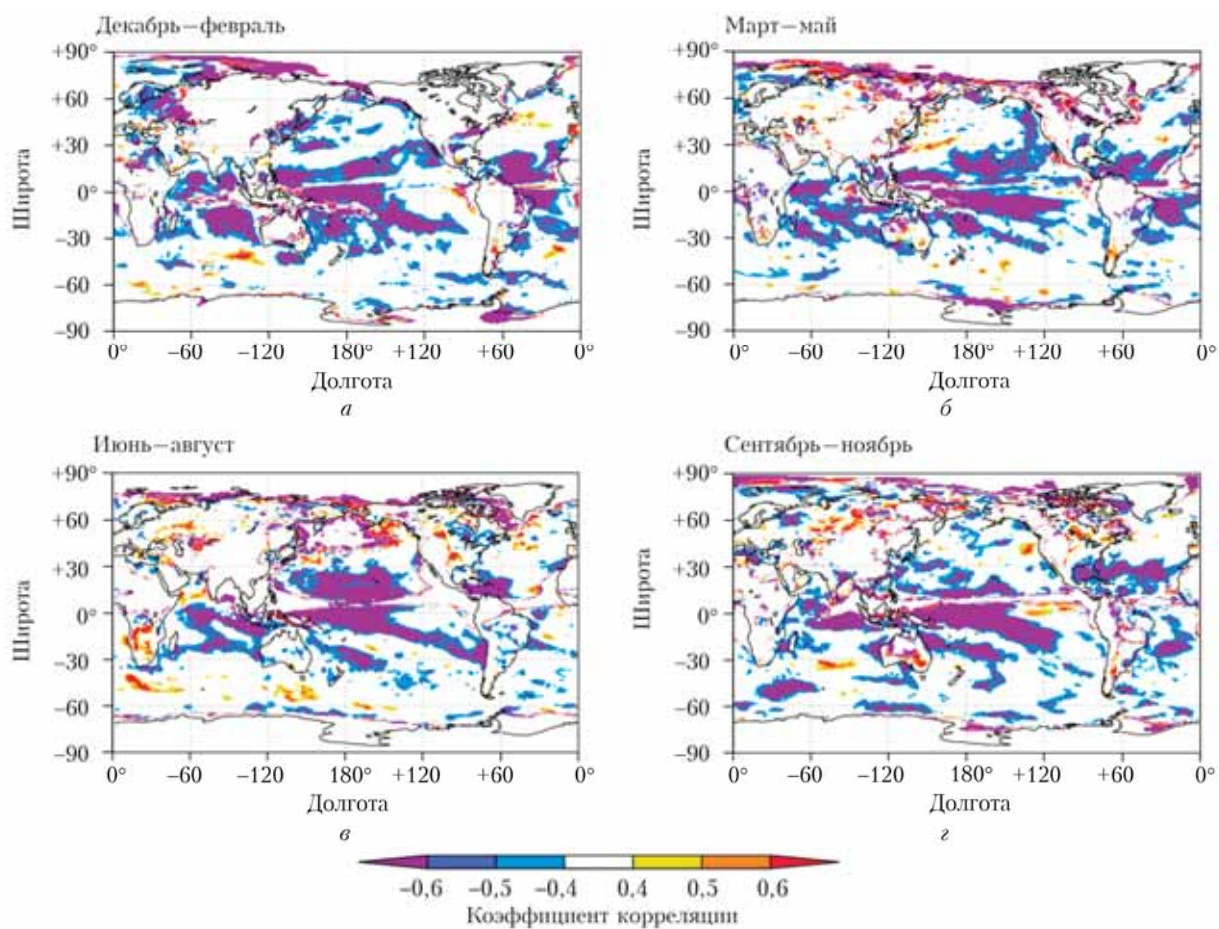
Рис. 5. Карты коэффициентов корреляций между среднесезонными значениями H_{\text{var}} и H_{\text{BL}} для зимы (а), весны (б), лета (в) и осени (г)
