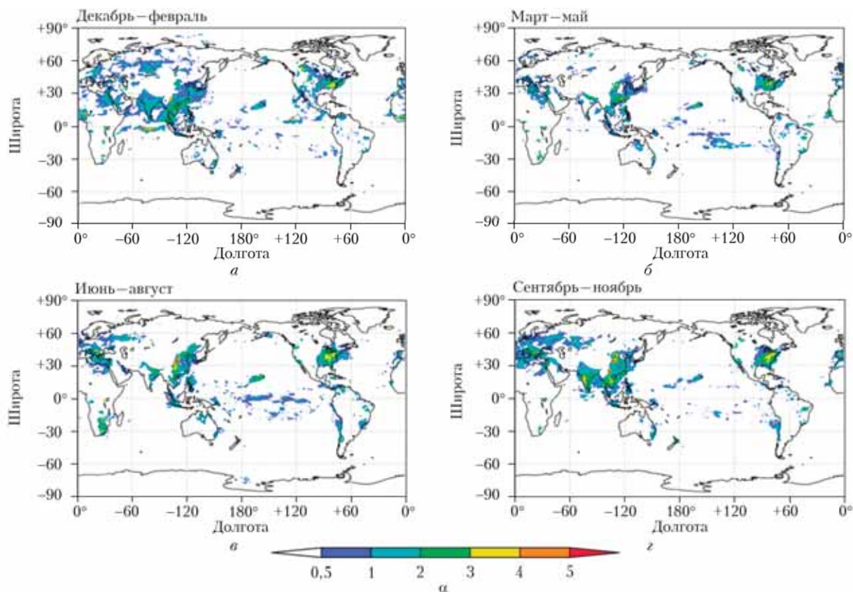
Рис. 9. То же, что и на рис. 8, но для коэффициента \alpha межгодовой линейной регрессии H_{SO_4} на H_{SO_2} для зимы (а), весны (б), лета (в) и осени (г)
