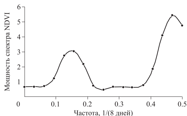
Рис. 2. Типичный вид спектра функции h(f) отклика NDVI на изменение LST (очаг, площадка № 10, 2010 г.).
