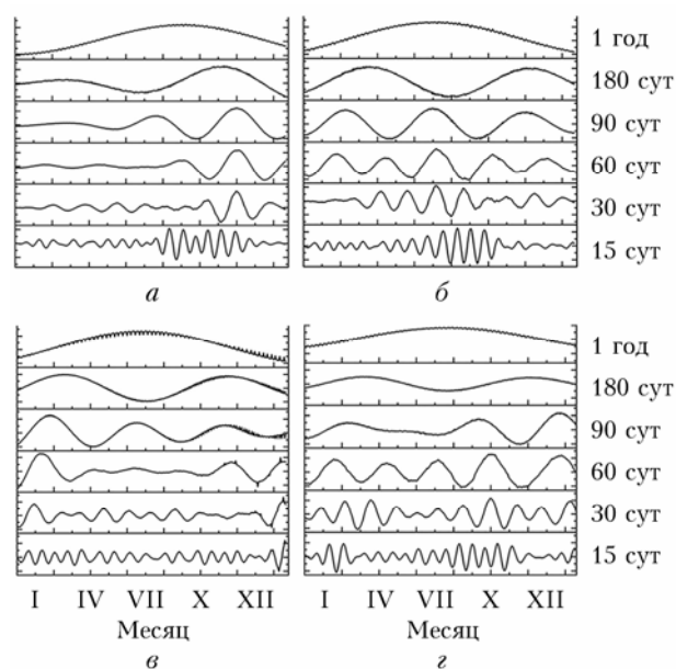
Рис. 4. Частотные характеристики результатов вейвлет-преобразования: a_{\text{ph}}(678) (а), TChl (б), b_{\text{bp}}(438) (в), a_{\text{CDM}}(438) (г), полученные по результатам моделирования для центральной части Азовского моря (AZ2) в 2019 г.
