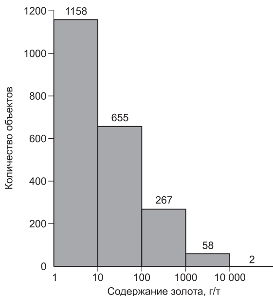
Рис. 3. Распределение штучных проб из рудопоявлений Яно-Колымской провинции по десятичным классам содержаний золота (всего 2140 объектов).
