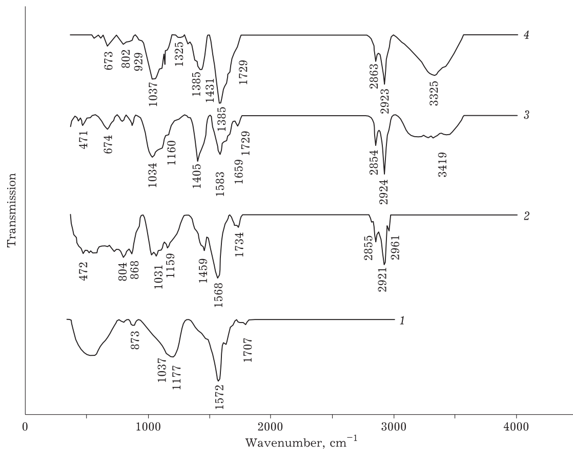
Fig. 1. FTIR spectra of samples: Taunite (1), CuMo/Taunite (2), CeCu/Taunite (3), CeMo/Taunite (4).
