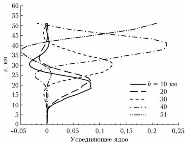
Рис. 3. Усредняющие ядра озонметра для озона. Диагональная ковариационная матрица озона
