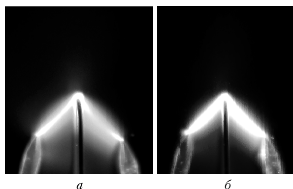
Рис. 3. Внешний вид разряда при U_p \sim 35 кВ, f = 8 Гц, p = 30 (а) и 110 торр (б), C = 30 (а) и 100 пФ (б). Время накопления 15 с (сложение 120 импульсов); высота кадра 1,8 см; камера Canon PowerShot SX60 HS в режиме накопления с экспозицией 15 с
