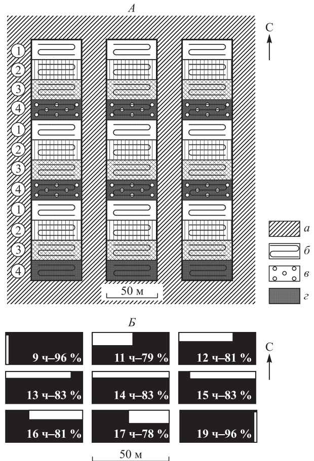
Рис. 6. Схема чересполосно-котловинной рубки (А) и дневной динамики площади затенения (%) котловин в день летнего солнцестояния на широте 55° (Б) в островных борах подзоны лесостепи.
