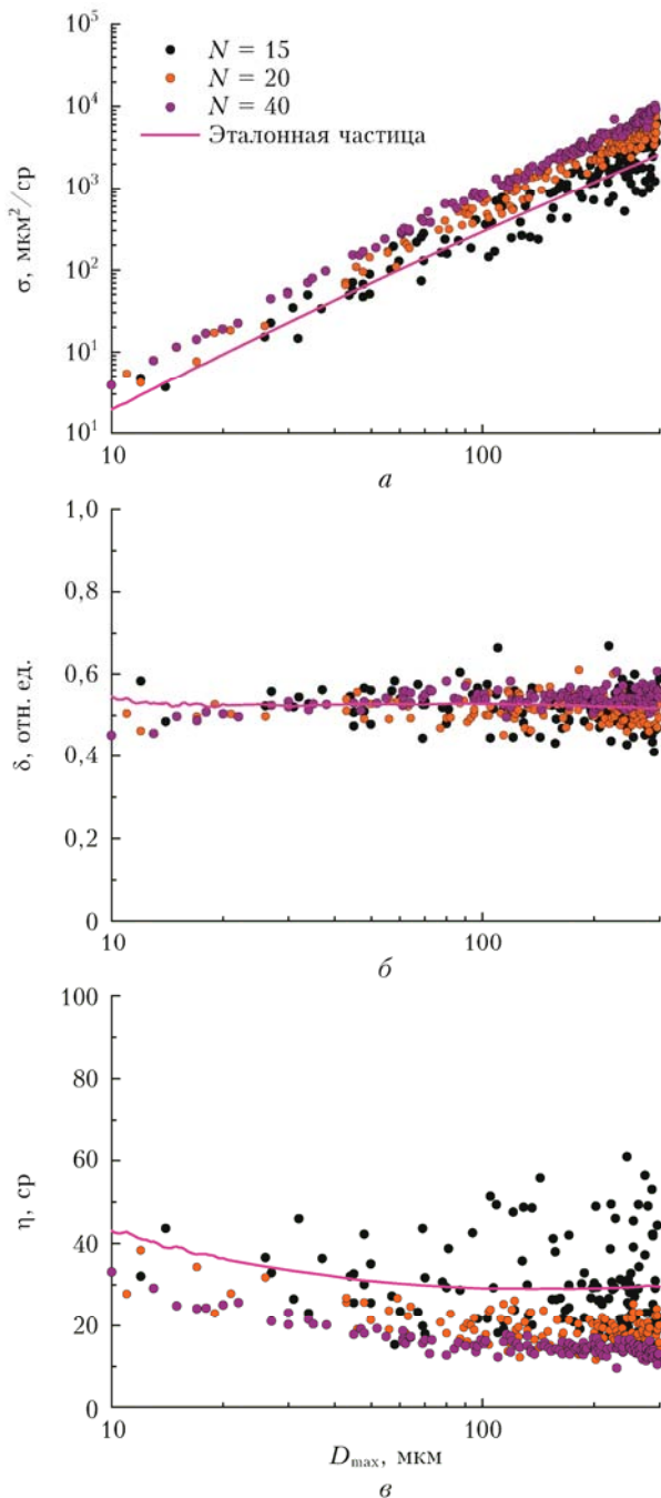
Рис. 3. Зависимости: дифференциального сечения рассеяния (а); линейного деполяризационного (б) и лидарного отношений (в) от D_{\max} для частиц произвольной формы; \lambda = 0,532 мкм (см. цветные рисунки на сайте http://iao.ru/ru/content/vol.37-2024/iss.10 )
