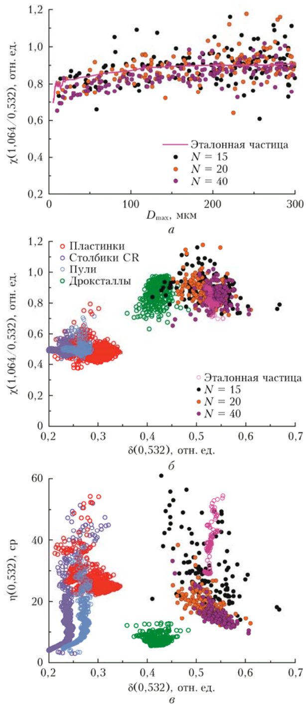
Рис. 4. Зависимости спектрального отношения от размера частицы (а) и линейного деполяризационного отношения (б); лидарного от линейного деполяризационного отношения (в) для частиц произвольной формы
