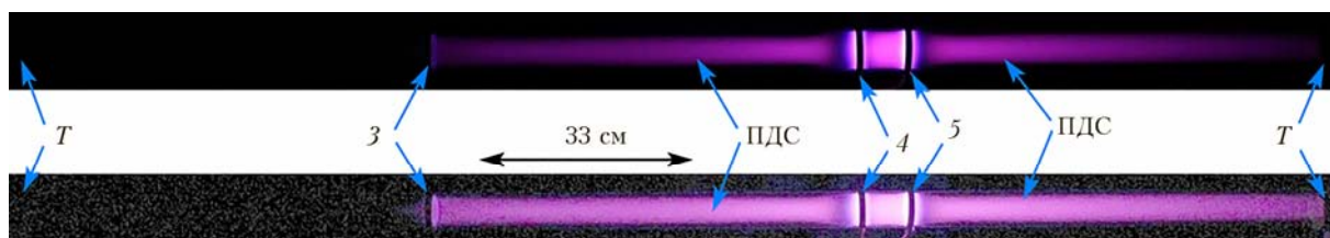
Рис. 6. Фотографии разряда, полученные с инициированием ПДС от плазмы емкостного разряда между электродами 4 и 5, на которые импульс напряжения подавался от генератора с напряжением U_1 при заземленных электродах 2 и 3 (электрод 2 не видно из-за слабой светимости разряда). Для верхнего снимка экспозиция 0,25 с; для нижнего светимость ПДС для тех же условий увеличена за счет коррекции яркости и контраста верхней фотографии (см. цветной рисунок на сайте http://iao.ru/ru/content/vol.37-2024/iss.04 )
