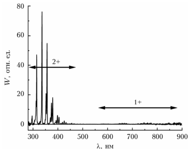
Рис. 7. Спектр излучения разряда в ЯО, полученный с помощью спектрометра HR2000 при p = 1,5 торр и задержке между запуском генераторов \approx 320 нс
