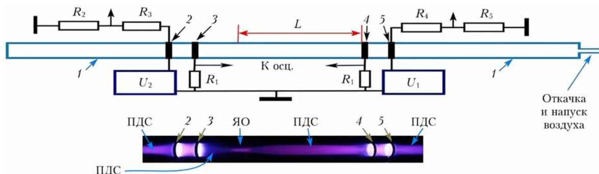
Рис. 2. Схема экспериментальной установки для изучения условий появления ЯО при встрече ПДС, инициируемых емкостным разрядом (вверху), а также фотография излучения ПДС (экспозиция 0,25 с) при давлении воздуха p = 1,5 торр с ЯО в виде цилиндра и свечения емкостного разряда между двумя парами электродов (внизу): 1 — кварцевая трубка; 2 — высоковольтный электрод, соединенный с генератором U_2 и делителем напряжения ( R_2-R_3 ); 3 — электрод, заземленный через шунт R_1 и соединенный с генератором U_2 ; 4 — электрод, заземленный через второй шунт R_1 и соединенный с генератором U_1 ; 5 — высоковольтный электрод, соединенный с генератором U_1 и делителем напряжения ( R_4-R_5 ); L — расстояние от левого края электрода 4 до места расположения в черном экране щели шириной 1 см, через которую излучение подавалось на спектрометр или фотоэлектронный умножитель (ФЭУ) (см. цветной рисунок на сайте http://iao.ru/ru/content/vol.37-2024/iss.04 )
