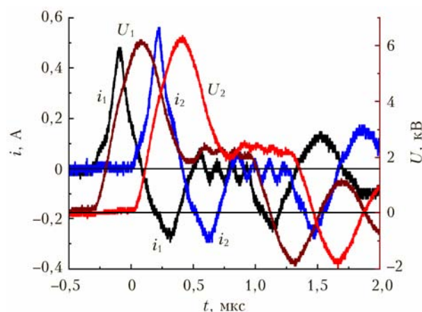
Рис. 3. Импульсы тока i_1 и i_2 , а также напряжения U_1 и U_2 при включении двух генераторов положительной полярности с задержкой между импульсами напряжения \approx 320 нс; p = 1,5 торр, U \approx 7 кВ (см. цветной рисунок на сайте http://iao.ru/ru/content/vol.37-2024/iss.04 )
