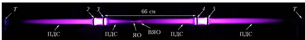
Рис. 4. Фотография разряда, полученная при включении двух генераторов с импульсами напряжения одинаковой полярности, p = 1,5 торр, U \approx 7 кВ, экспозиция 1 с: 2, 5 — высоковольтные электроды; 3, 4 — заземленные электроды. Здесь и далее T — торцы кварцевой трубки; ВЯО — вторая ЯО (см. цветной рисунок на сайте http://iao.ru/ru/content/vol.37-2024/iss.04 )
