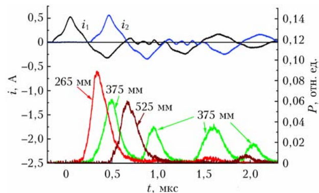
Рис. 5. Импульсы тока i_1 и i_2 , а также сигналы с ФЭУ при включении двух генераторов положительной полярности с задержкой 320 нс. Расстояния L от левого края электрода 4 до правого края щели шириной 0,5 см в черном экране, который устанавливался на поверхности кварцевой трубки, составляли 265, 375 и 525 мм. Световод ФЭУ располагался напротив центра щели; p = 1,5 торр, U \approx 7 кВ; P — мощность излучения (см. цветной рисунок на сайте http://iao.ru/ru/content/vol.37-2024/iss.04 )
