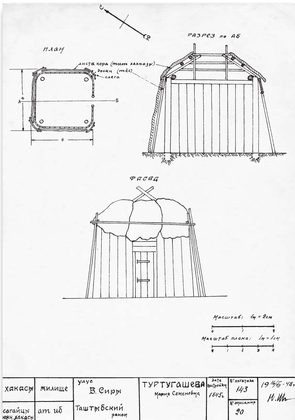
Рис 1. Жилище хакасов ам иб (По: Шибеева Ю.А. Чертежи по жилищу хакасов (55 чертежей), ХакНИИЯЛИ. Рук. фонд. № 352 (приложение)).
