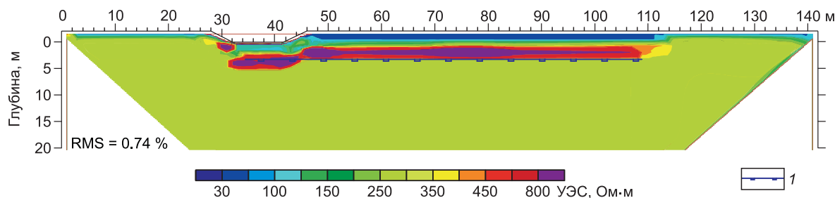
Рис. 3. Результат инверсии модельных данных с закрепленной границей:
