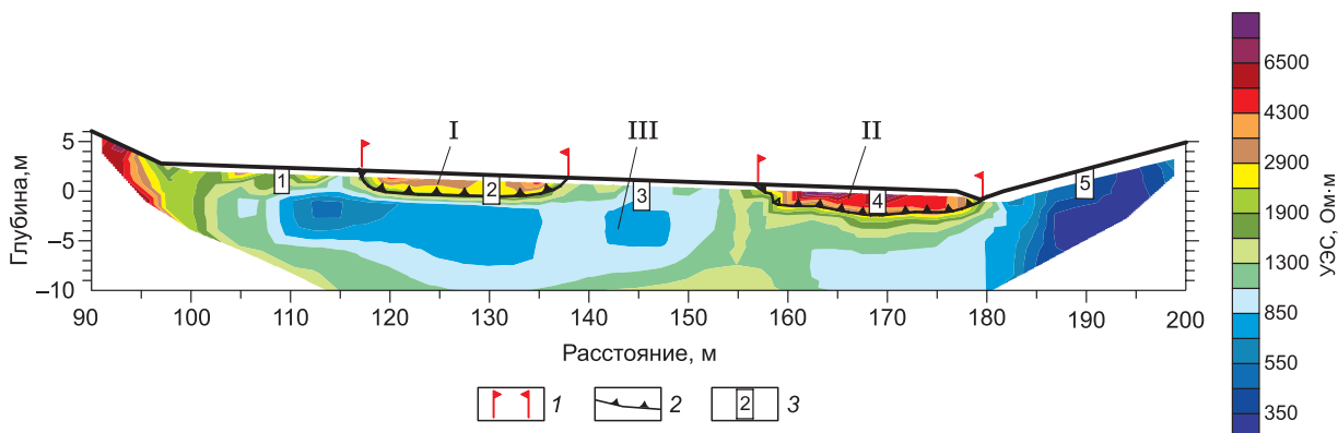
Рис. 8. Геоэлектрический разрез долины по данным ЭТ в Приморском хребте, Прибайкалье.
