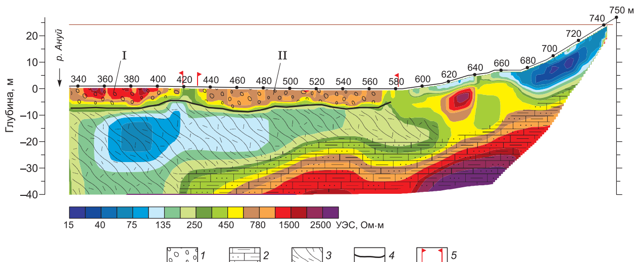
Рис. 7. Геоэлектрический разрез через долину р. Ануй, Алтай.
