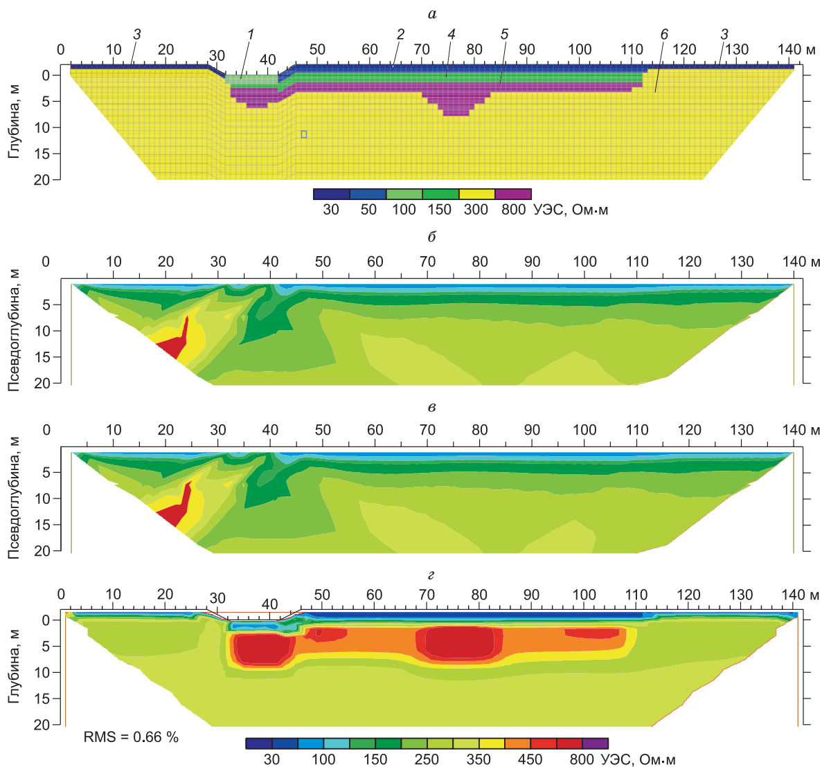
Рис. 2. Физико-геологическая (геоэлектрическая) модель долины реки (а), разрез наблюдаемых кажущихся УЭС (б), разрез расчетного кажущегося УЭС (в), результат 2-D инверсии модельных данных (г):
