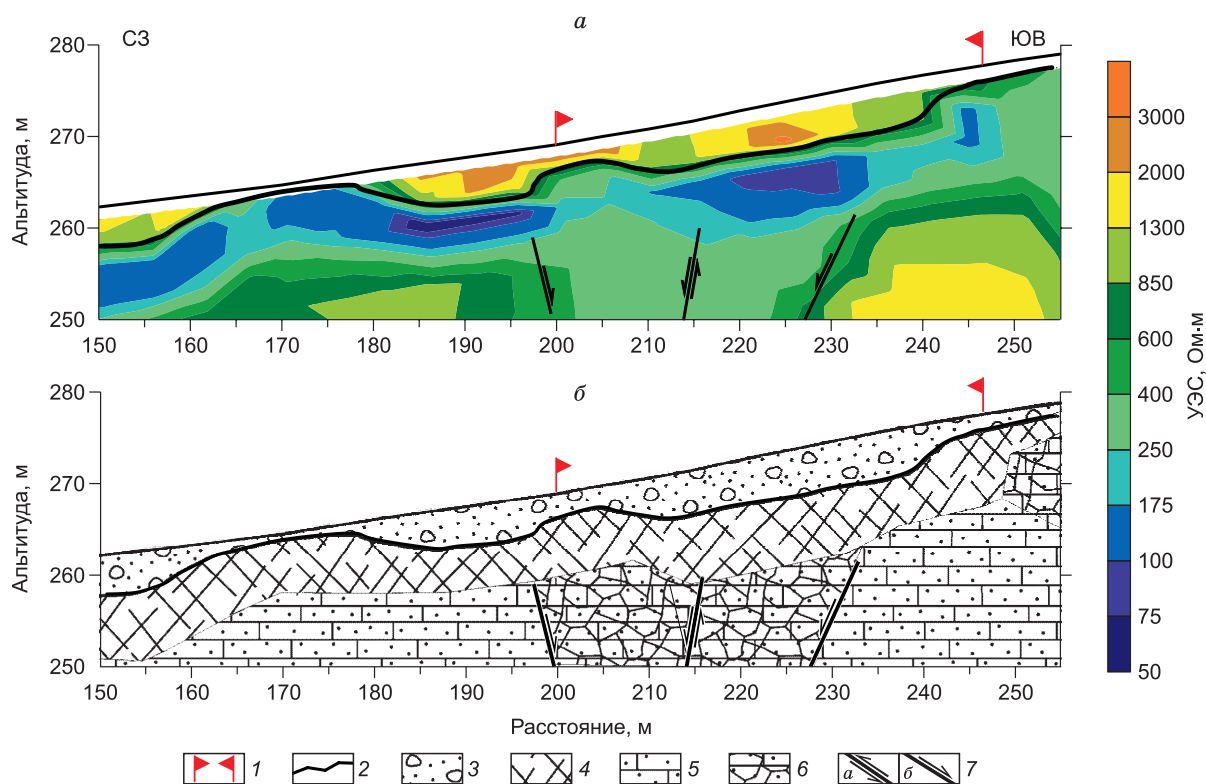
Рис. 5. Геоэлектрический разрез вдоль разведочной траншеи (а) и его интерпретация (б) с учетом геологических данных.
