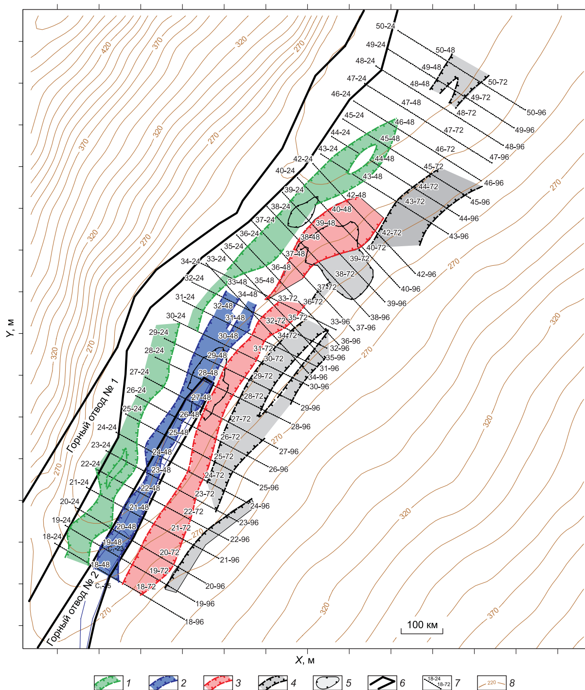
Рис. 6. Схема распределения аллювиальных отложений русловой фации по геофизическим данным.
