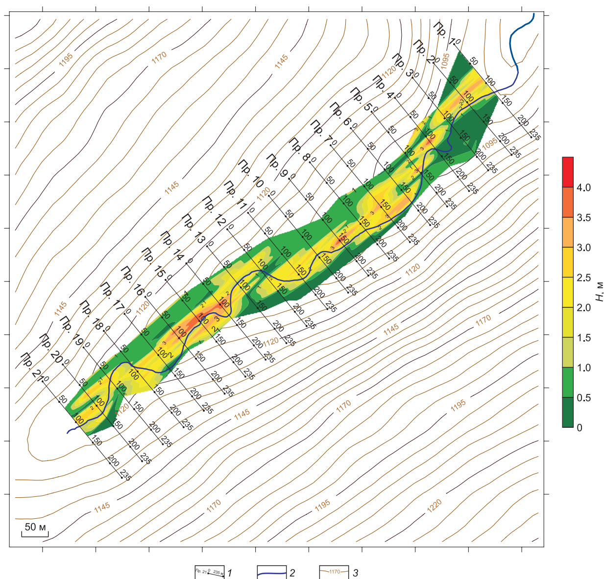
Рис. 9. Карта мощности рыхлых отложений по данным электротомографии, Прибайкалье:
