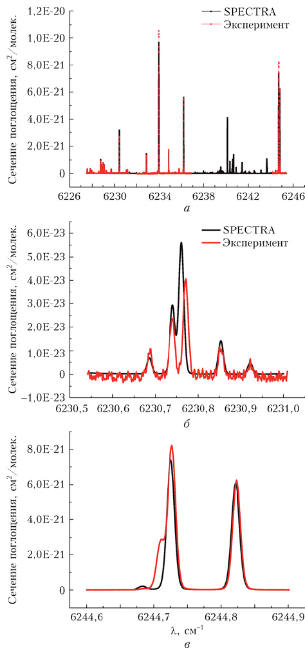
Рис. 3. Экспериментальные спектры \text{H}_2\text{S} в сравнении с данными системы SPECTRA (а) и фрагменты этих спектров (б, в) при P = 0,00266 \text{ атм} (см. цветной рисунок на сайте http://iao.ru/ru/content/vol.37-2024/iss.01 )
