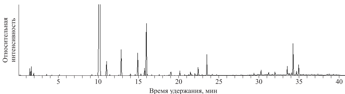
Рис. 2. Хроматограмма летучих веществ (на примере КС) – паровая фаза прободобор.
